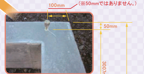
100mm ※50mmではありません。
