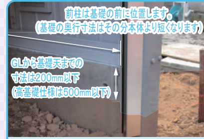
前柱とシャッターレールは地中に埋め込みます。
