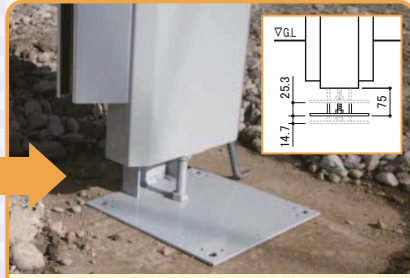
アジャスターで多少の高さ調整が出来ます。 調整範囲は374~414mmです。
